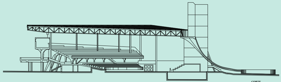
CORTE
