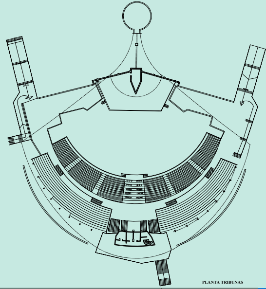
PLANTA TRIBUNAS
